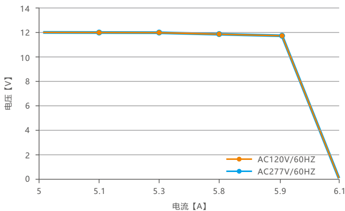
过载曲线
