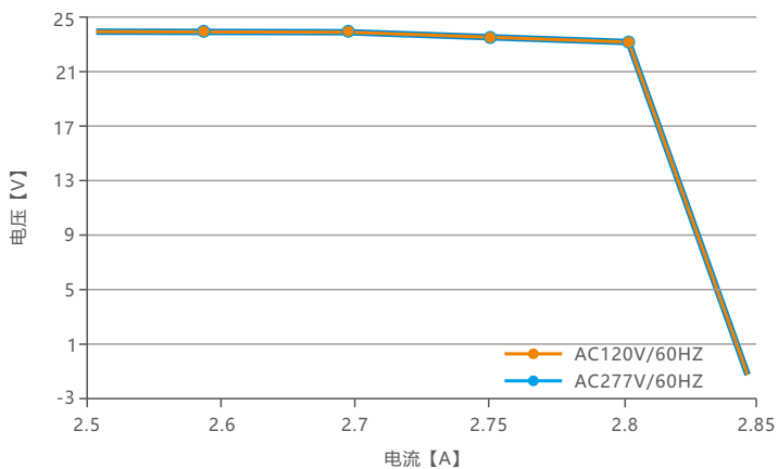
过载曲线
